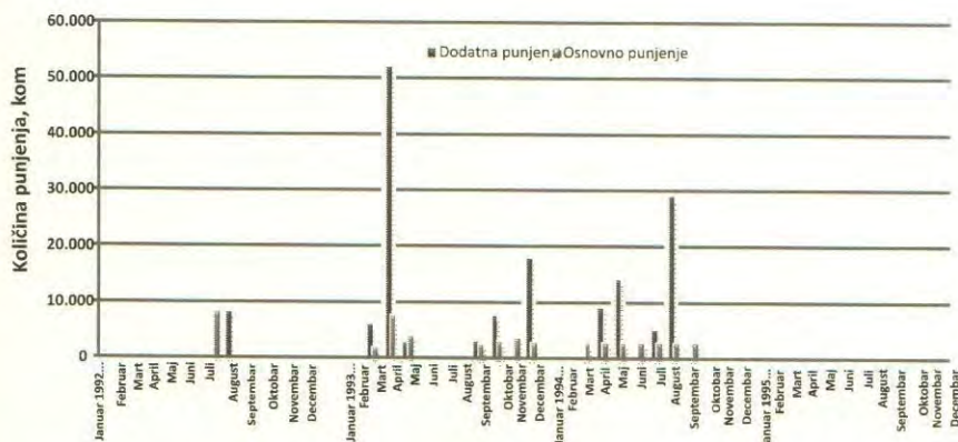
Fig. 20. Količina uvezenih osnovnih i dodatnih punjenja za minobacačku municiju 120 mm u periodu rata 1992-1995. godine
