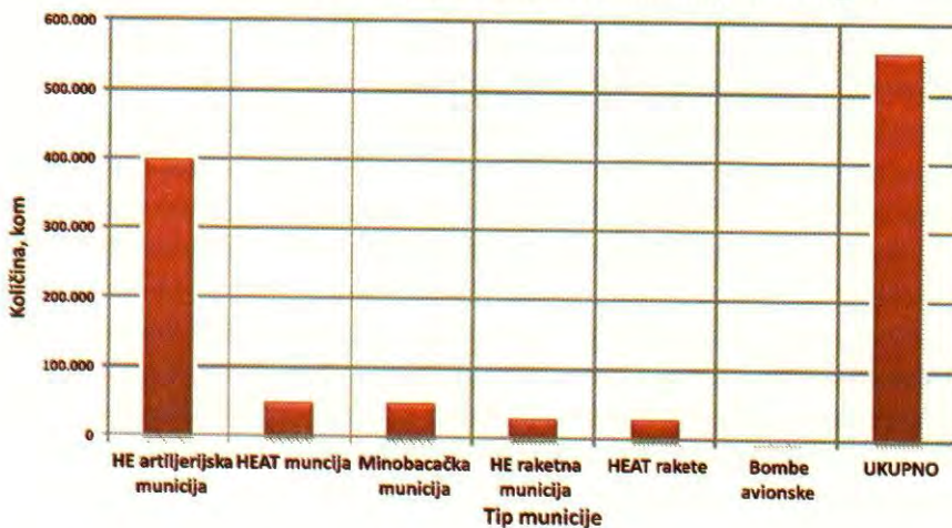
Fig. 3. Kapacitet proizvodnje municije velikog kalibra po tipovima municije u 1990. godini u tvornici “Pretis”
