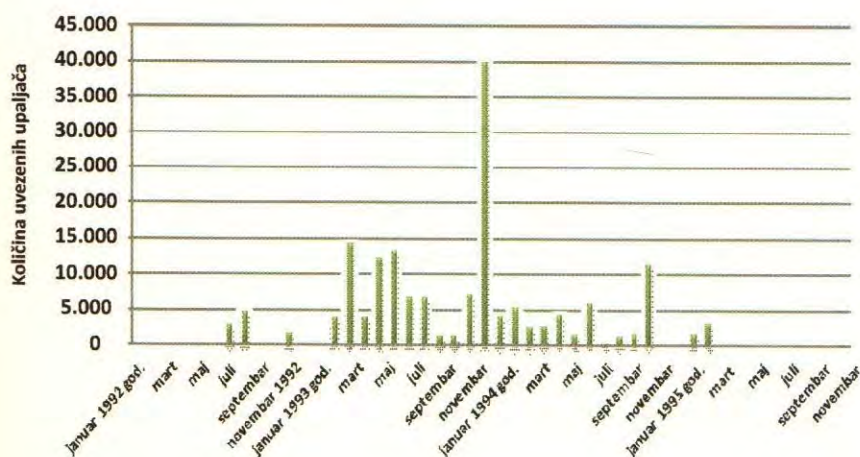
Fig. 18. Struktura uvoza upaljača za municiju velikog kalibra iz SR Jugoslavije u periodu rata 1992-1995. godine (ukupno uvezeno 169.501 komada)
