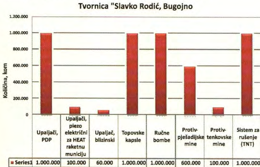
Fig. 6. Kapacitet proizvodnje upaljača za municiju velikog kalibra, ručnih bombi i mina u 1990. godini u tvornici "Slavko Rodić", Bugojno
